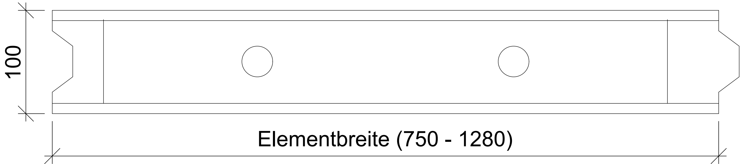
Elementschnitt (VGE)
