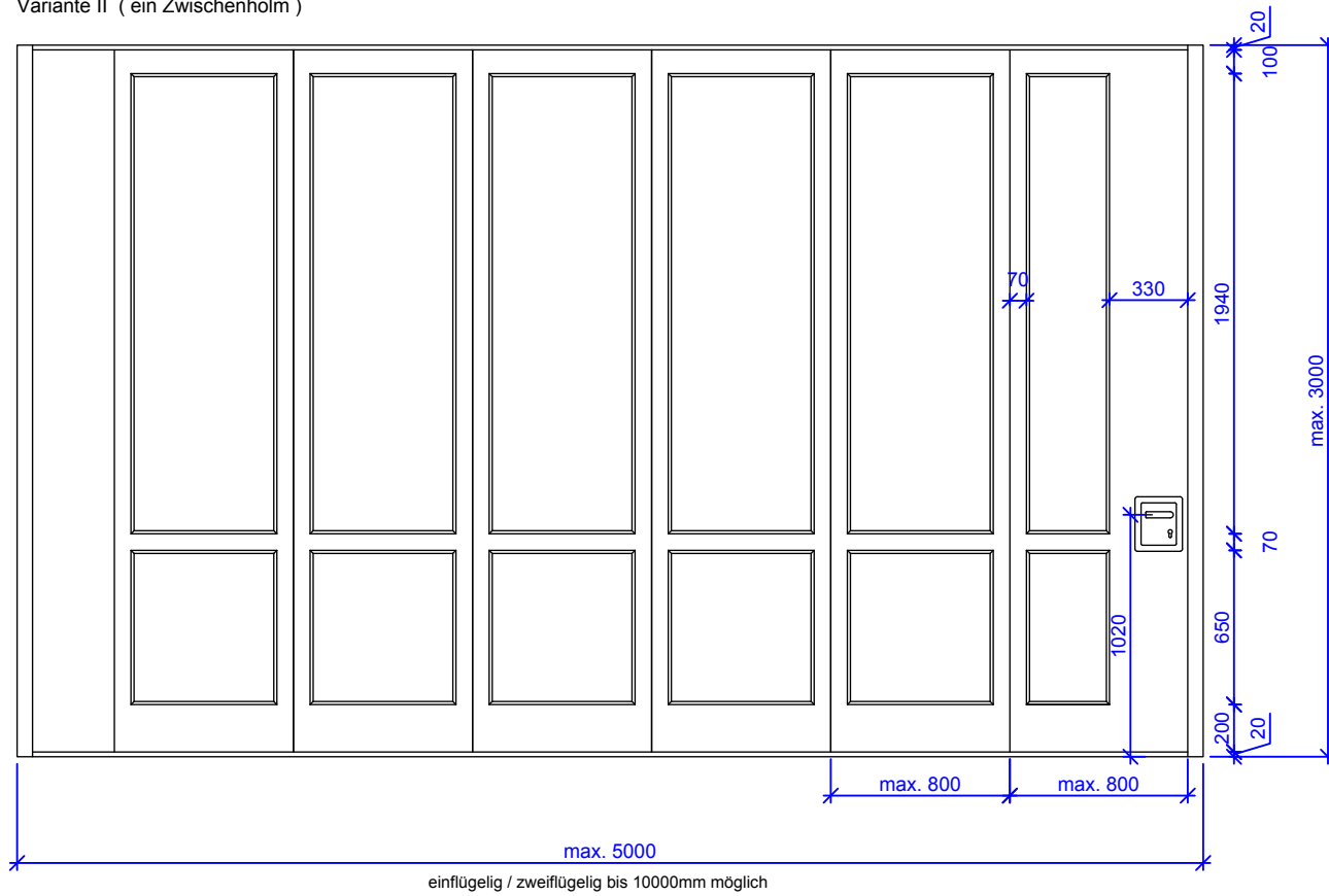
Variante II ( ein Zwischenholm )
