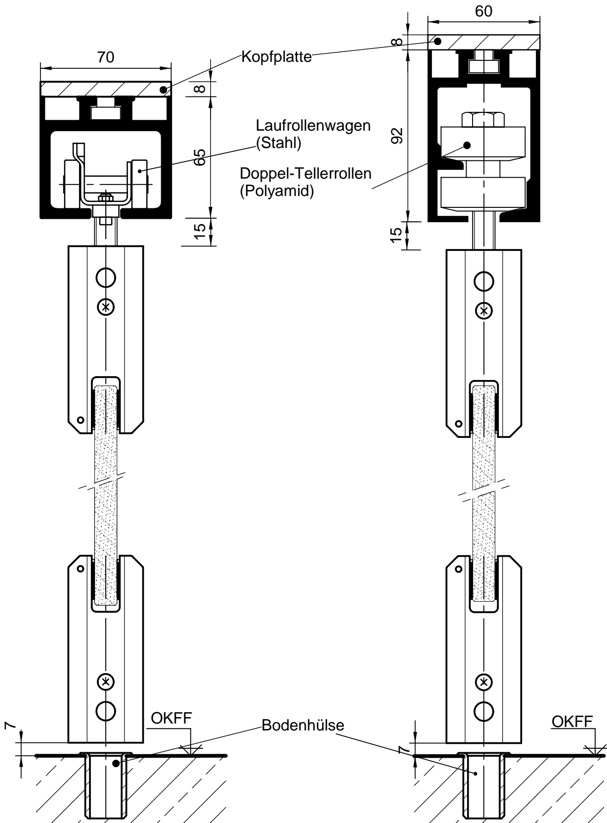
Alu- Laufschiene Typ L
